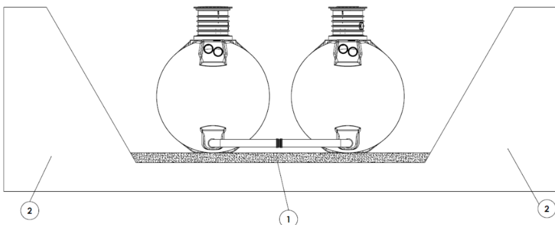
① Bettung ② Anstehender Boden
